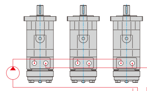
並列接続
