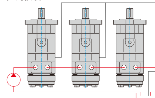
直列接続 ドレン配管
